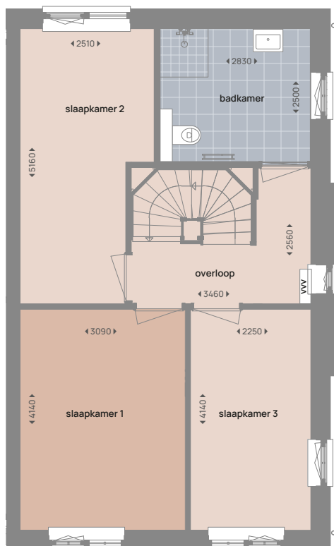
Eerste verdieping
